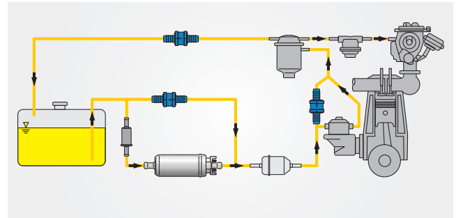
Uygulama örneği: Anahtarlanabilir elektrikli ilave pompası olan karbüratörlü motor
